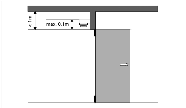
Abb. 3: Drehflügeltüren bis max. 3 Meter lichte Breite
