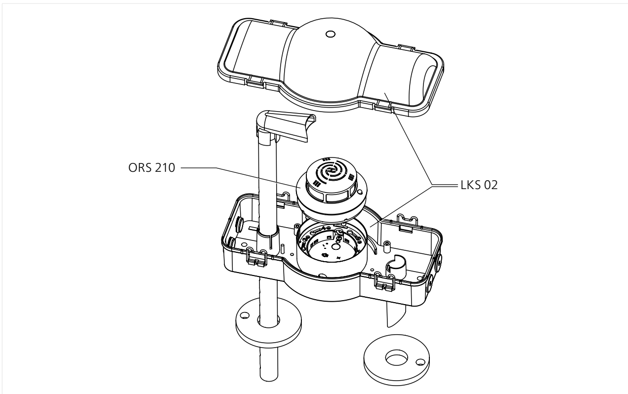
Abb. 1: Lüftungs-Rauchscharter-System LRS 01
