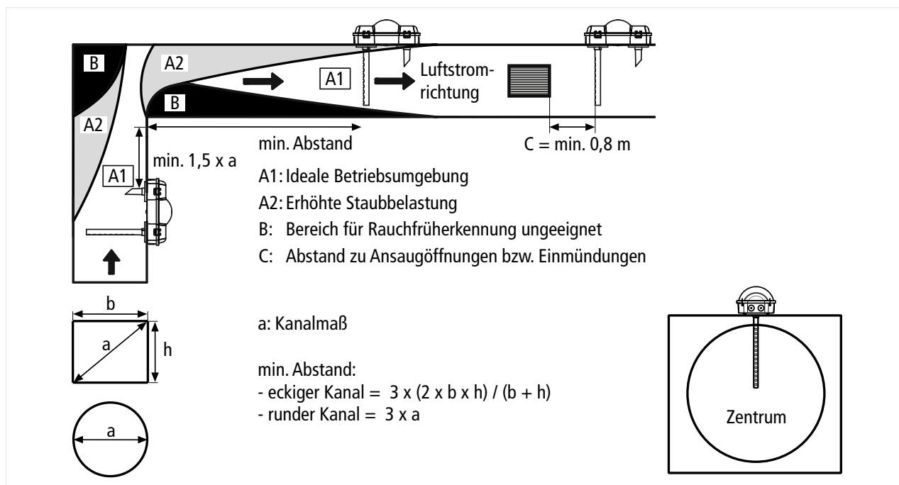
Abb. 2: Projektierungsübersicht
