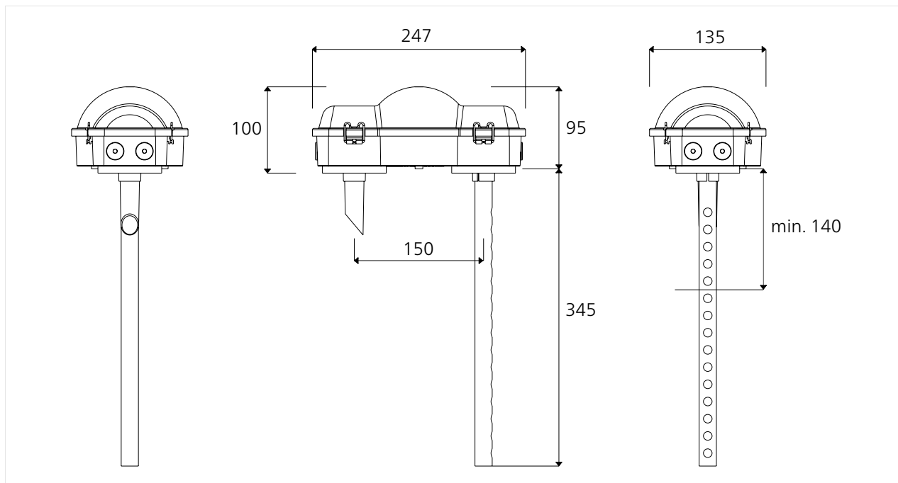
Abb. 3: Maßbild
