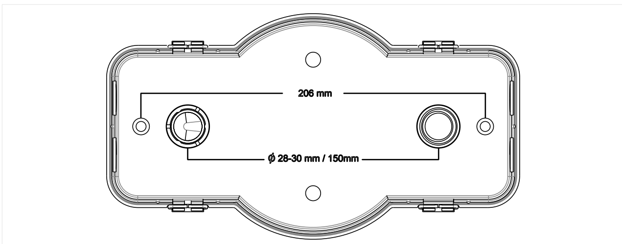
Abb. 5: Bohrmaße
