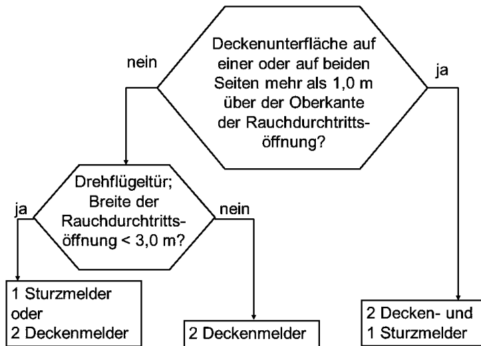
Bild 4: Entscheidungsdiagramm
