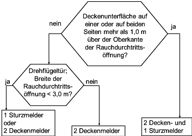
Bild 4: Entscheidungsdiagramm
