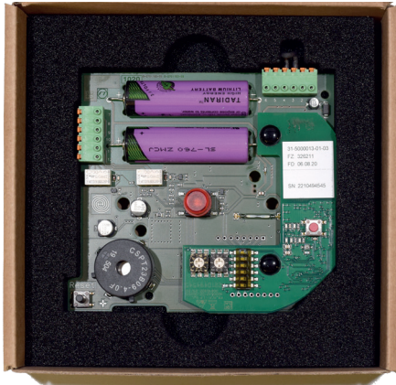
Abb. 1: Austauschmodul (Auslieferungszustand)
