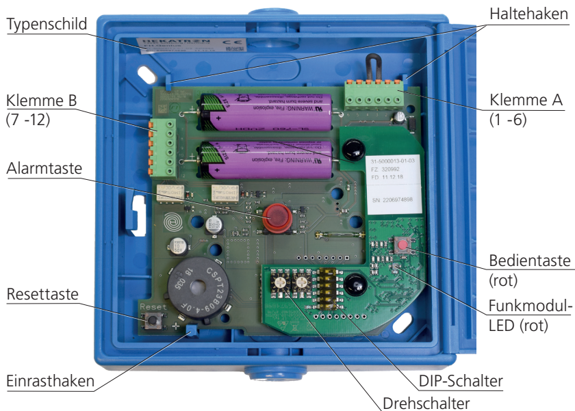
Abb. 2: Genius Funkhandtaster
